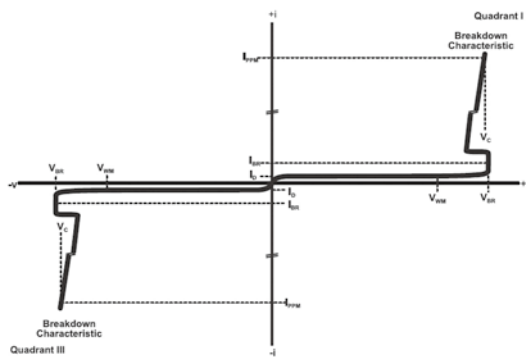
图 PTVS的V/I曲线
