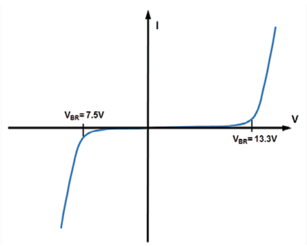
图7. CDSOT23-SM712 I/V特性
