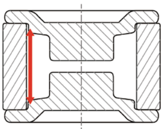
图 基于传统工艺的GDT的内部截面
