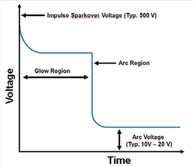
图10. GDT特性波形
