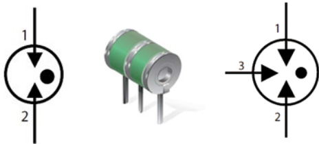
图 三电极气体放电管及其符号
