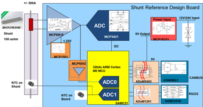
图 方案功能框图
