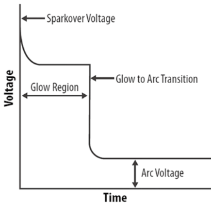
图 GDT特性曲线
