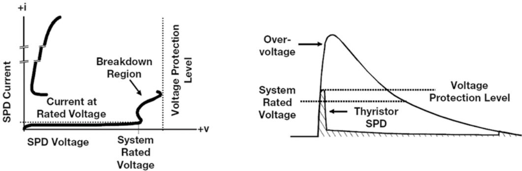
图 TISP®器件切换浪涌能量V/I曲线及电压限制波形图
