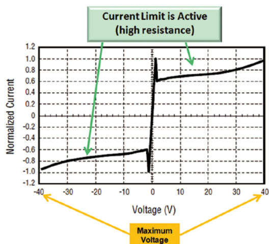
图 TCS™ 保护器件的V/I曲线
