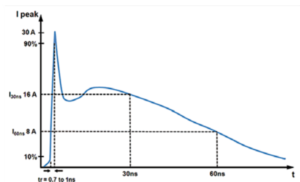
图1. IEC61000-4-2 ESD波形(8 kV)
