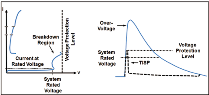
图9. TISP切换特性和电压限制波形
