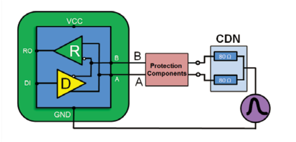
图4. 半双工RS-485器件的耦合/解耦网络
