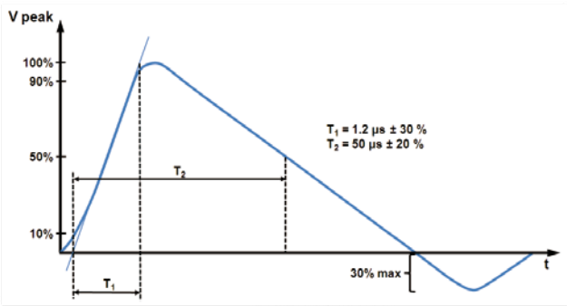
图3. IEC61000-4-5电涌1.2/50 波形
