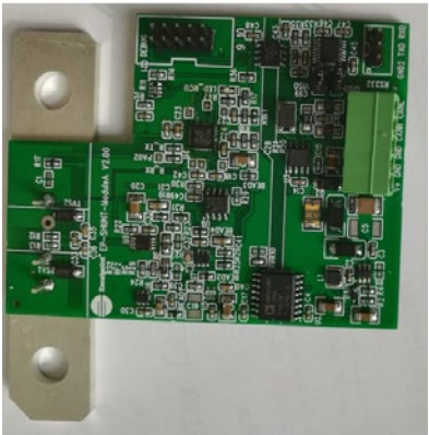
图 SHUNT分流器电流检测方案PCBA
