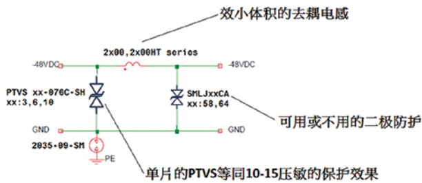
使用PTVS 之48V DC 防护电路
