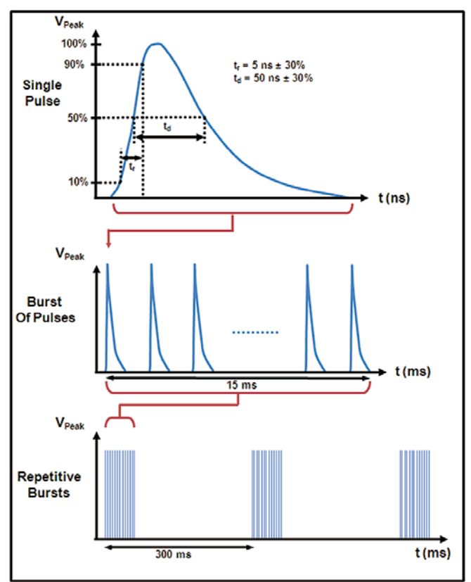
图2. IEC61000-4-4 EFT 50 负载波形
