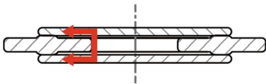
图 基于FLAT®皱接工艺GDT的内部截面
