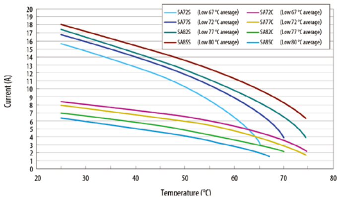
图 不同温度下动作曲线图 (以SAXXX系列为例)
