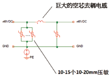
传统的48VDC 防护电路
